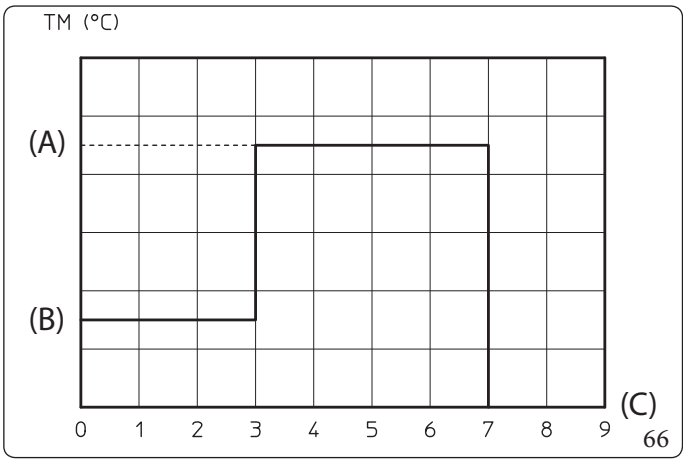
Leyenda (Fig. 66): (A) - Ajuste superior (B) - Ajuste inferior (C) - Días TM - Temperatura de impulsión
