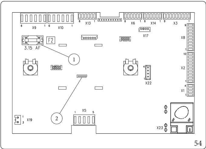
Leyenda (Fig. 54): 1 - Fusible 3,15 rápido de 250 V Tipo F 2 - Memoria extraíble de color gris (A19)
