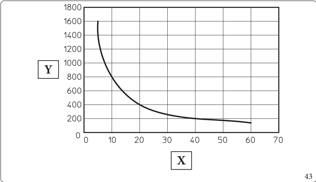
Leyenda (Fig. 43): X - Dureza total del agua °F Y - Litros agua sistema
