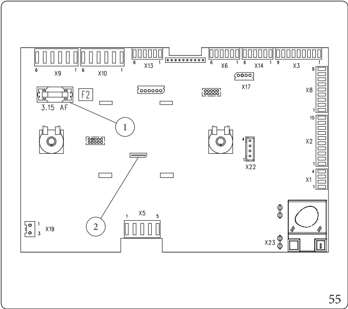
Leyenda (Fig. 55): 1 - Fusible 3,15 rápido de 250 V Tipo F 2 - Memoria extraíble de color gris (A19)
